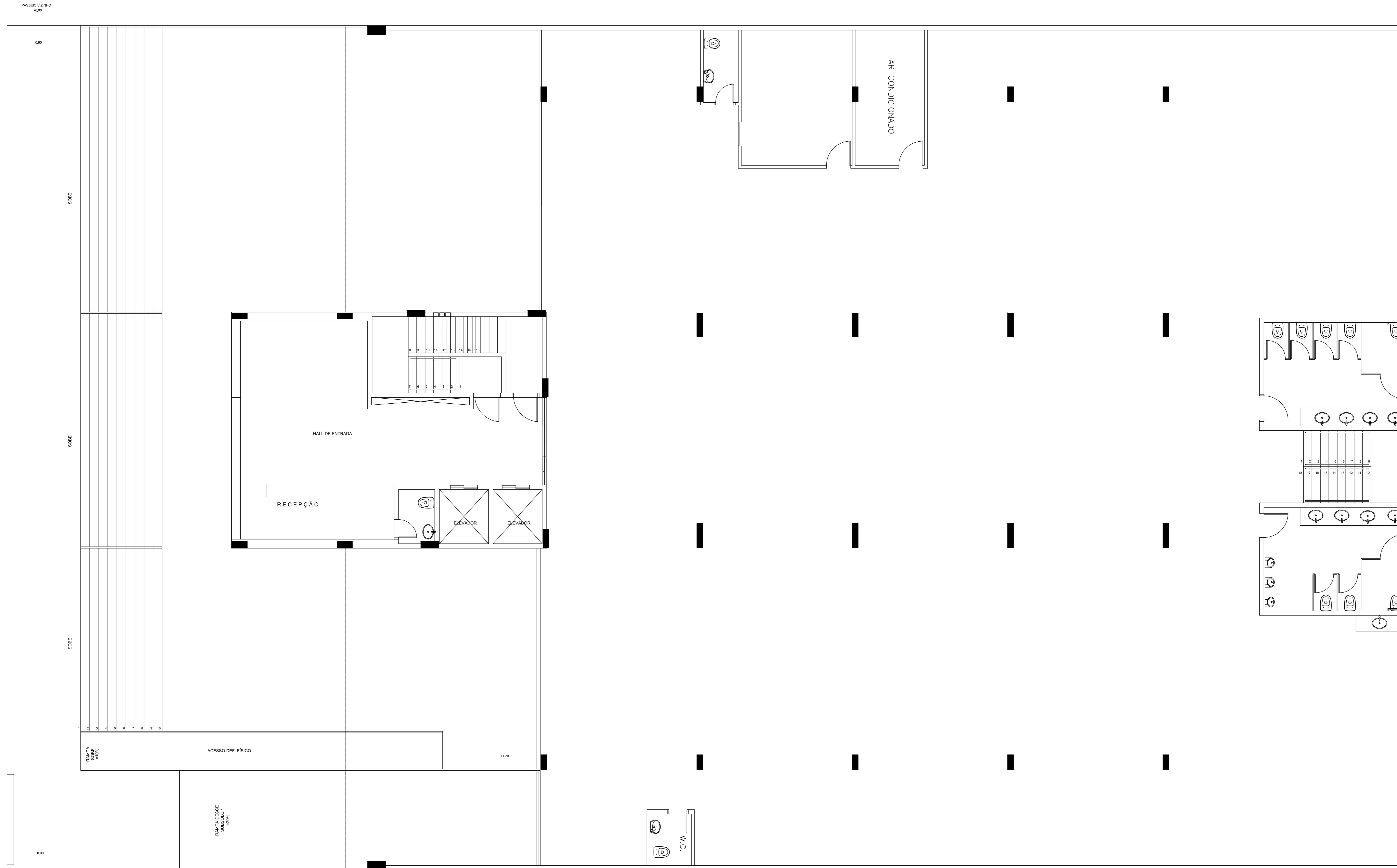
PLANTA BAIXA TÉRREO esc.: 1/50
