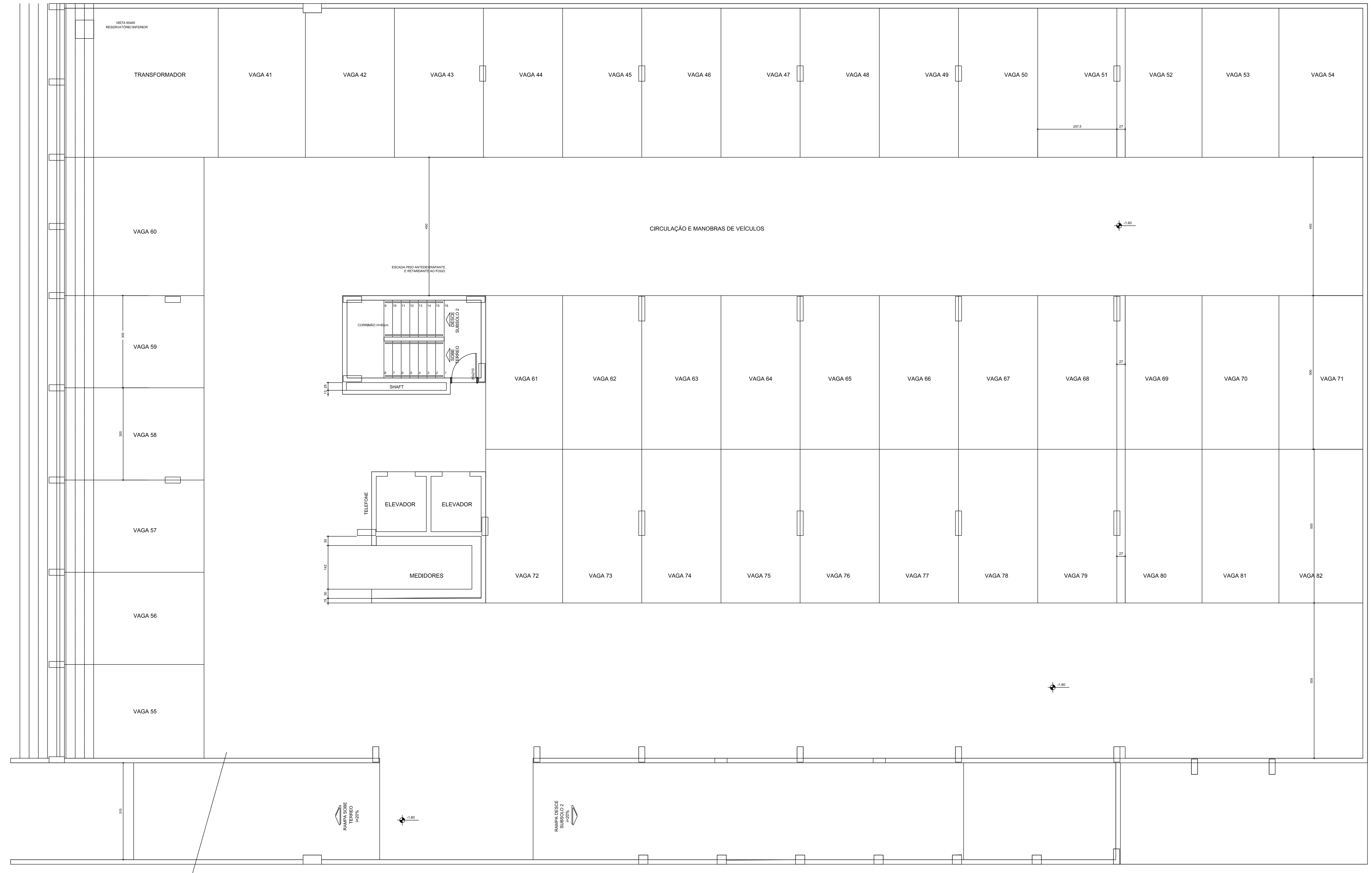
PLANTA BAIXA SUBSOLO 1 esc.: 1/50
