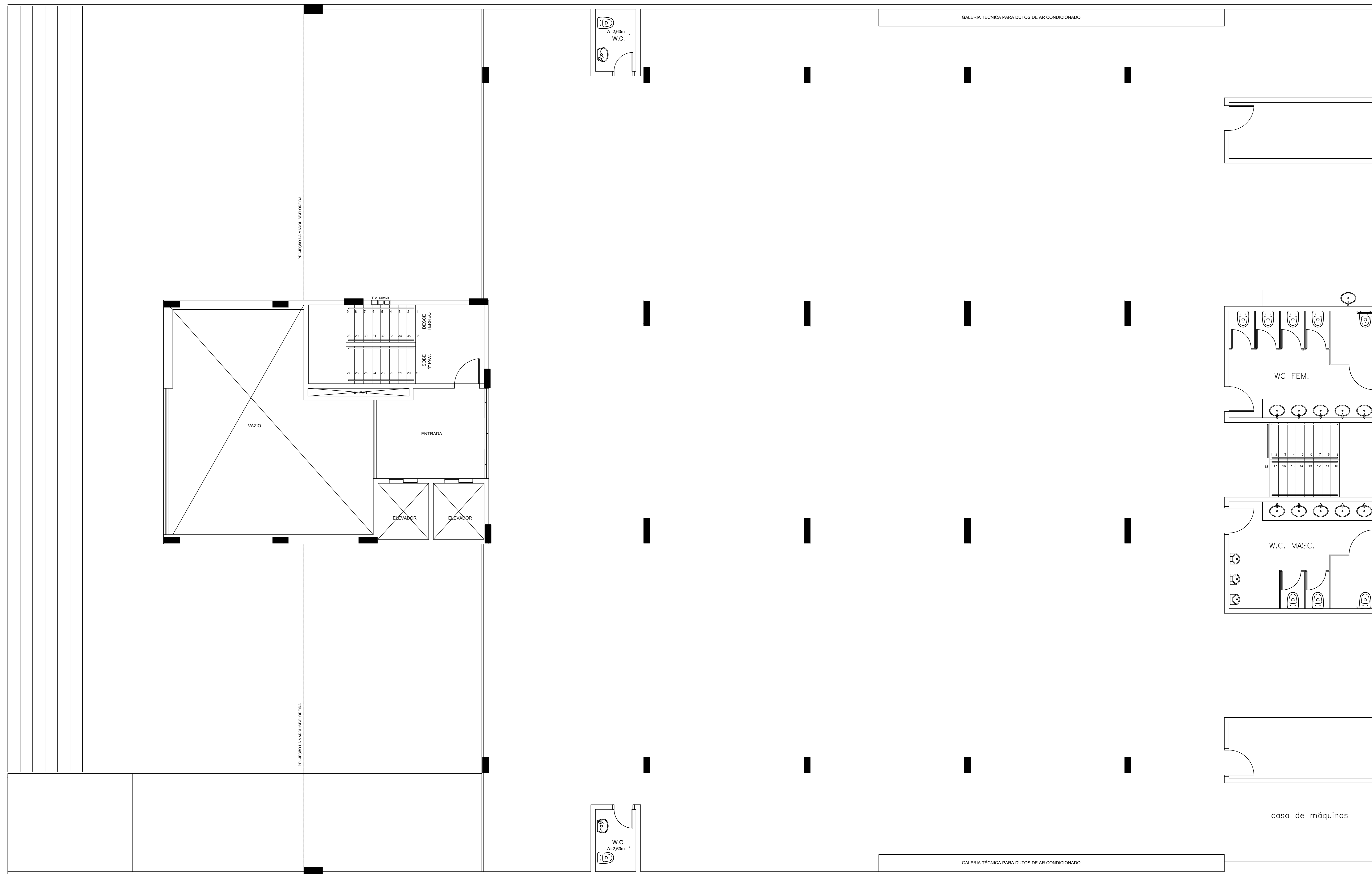
PLANTA BAIXA MEZANINO esc.: 1/50
